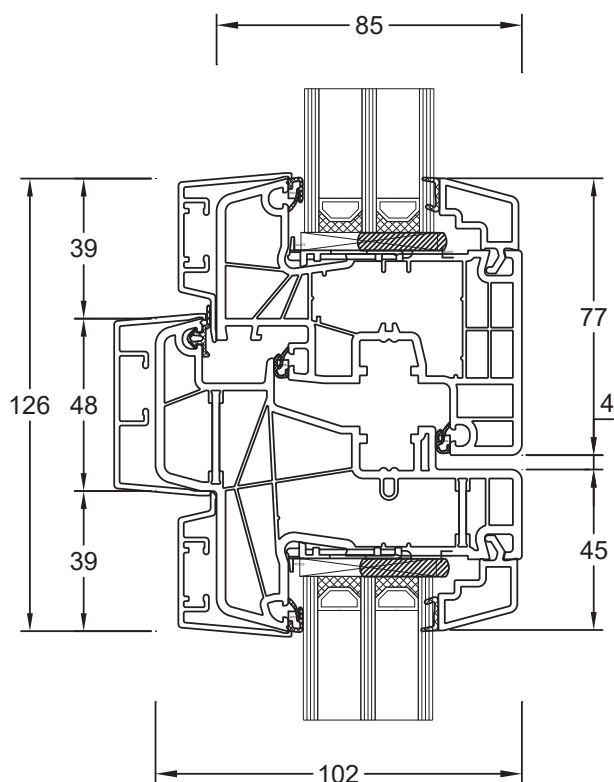
Stulpflügel 080x89/S 12633+ S12647 Flügel Classic 180x20/ S12631
