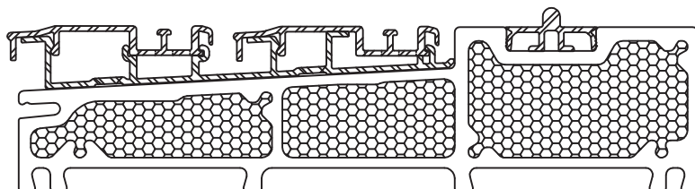
Schwelle PREMIUM / GFK / barrierefrei + Trittschutz 277107/277106
