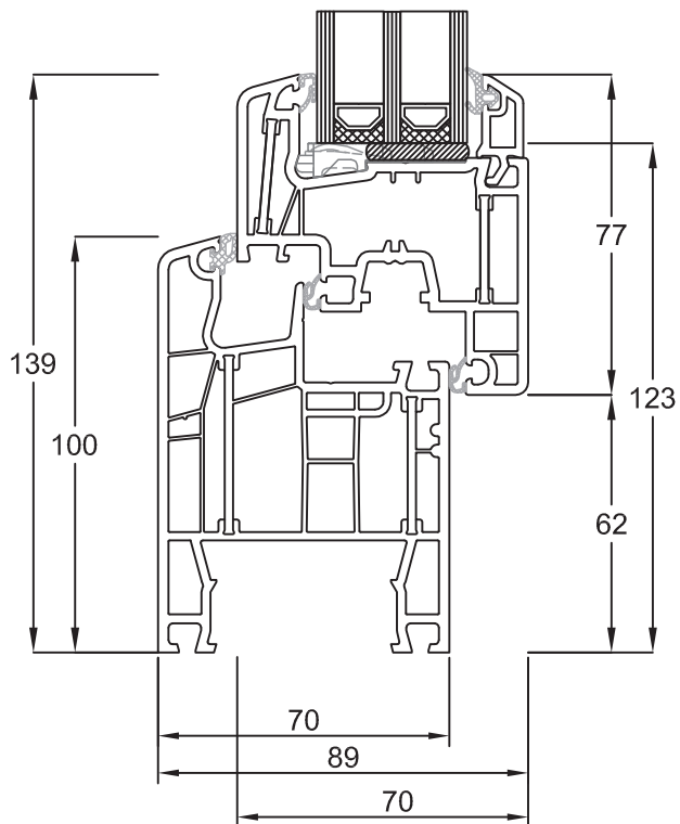
Blendrahmen 050x04 Flügel Classic 050x20
