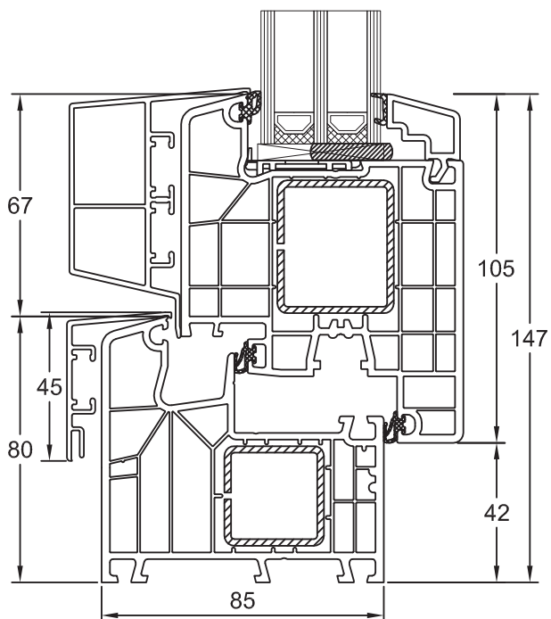
Blendrahmen 180x05/ S12628 Flügel Classic 180x30/ S12640
