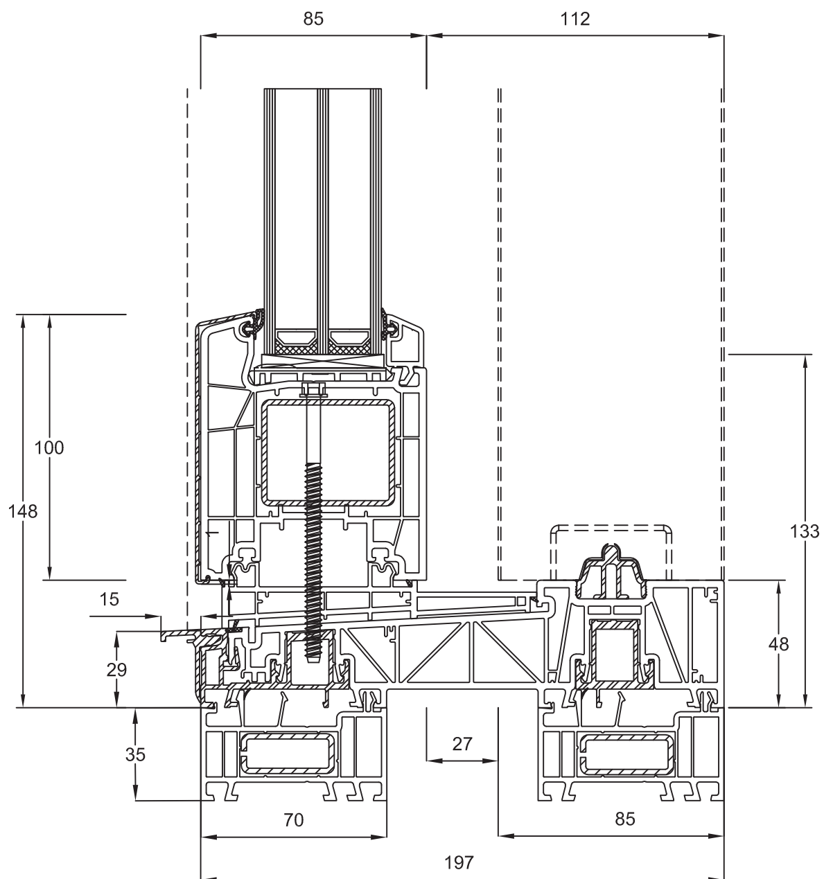
Schwelle Standard 277260 Flügel 170x81 STV 140205
