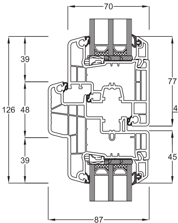
Stulpflügel 150x68 Flügel Classic 150x20
