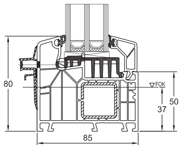
Blendrahmen 180x05 Einlegeschwelle FIX
