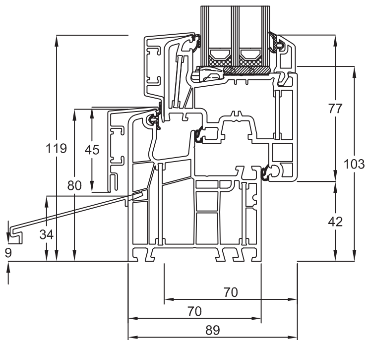
Blendrahmen 050x03 Flügel Classic 050x20 Wetterschenkel S12833
