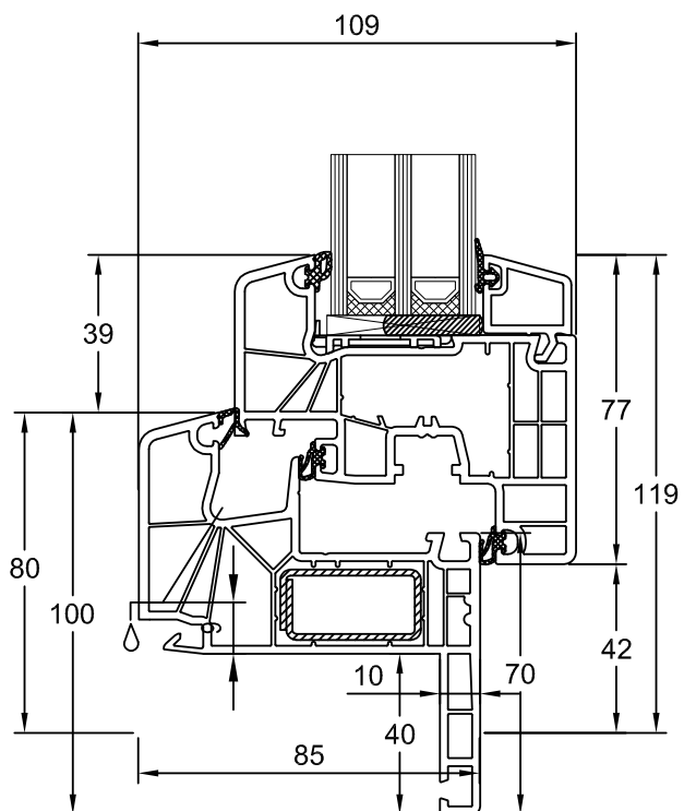
Blendrahmen 180x15 Flügel Classic 180x20
