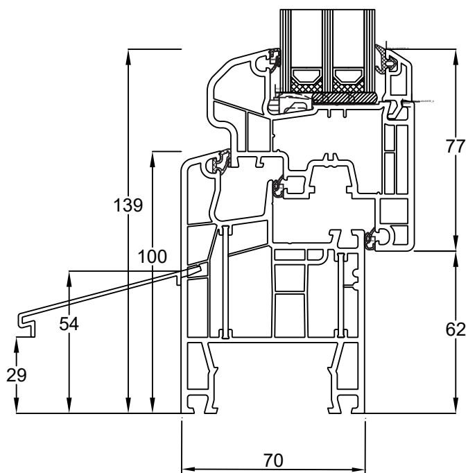
Blendrahmen 050x04 Flügel hfv 150x26 Wetterschenkel S12833
