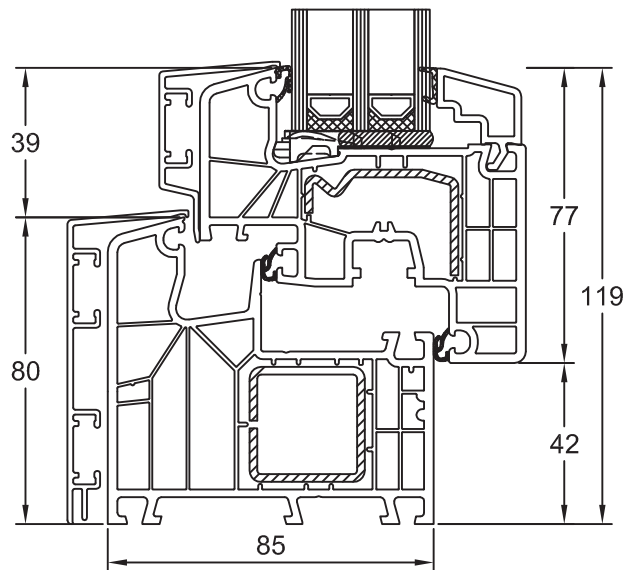
Blendrahmen 180x05/ S12929 Flügel Classic 180x20/ S12631
