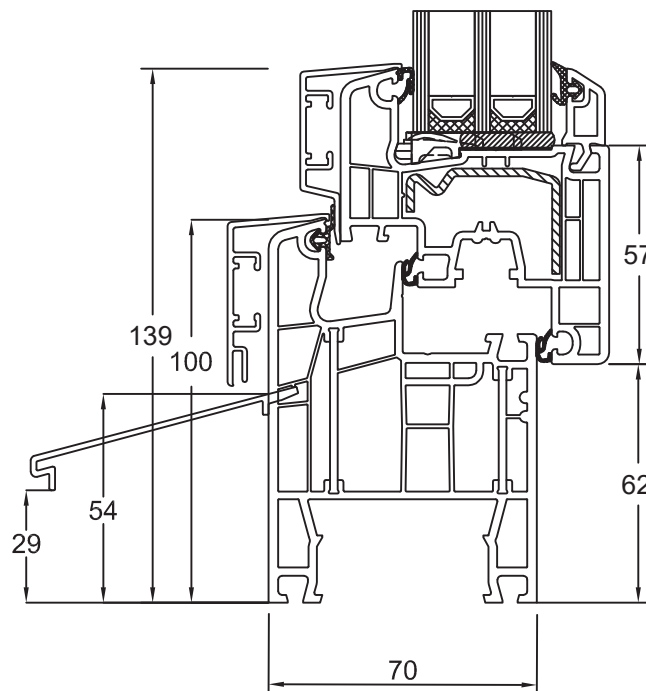
Blendrahmen 050x04 Flügel Classic 150x20 Wetterschenkel S12833
