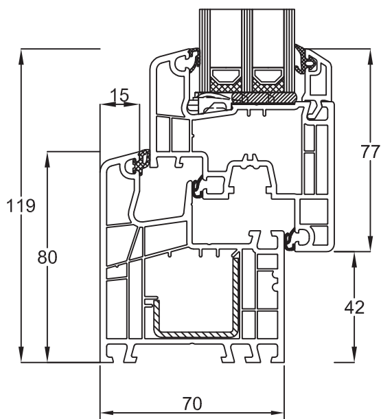
Blendrahmen 150x03 Flügel Classic 150x20
