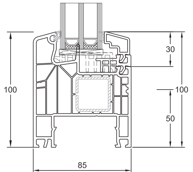
Blendrahmen 180x04 Flügel HFV 180x26
