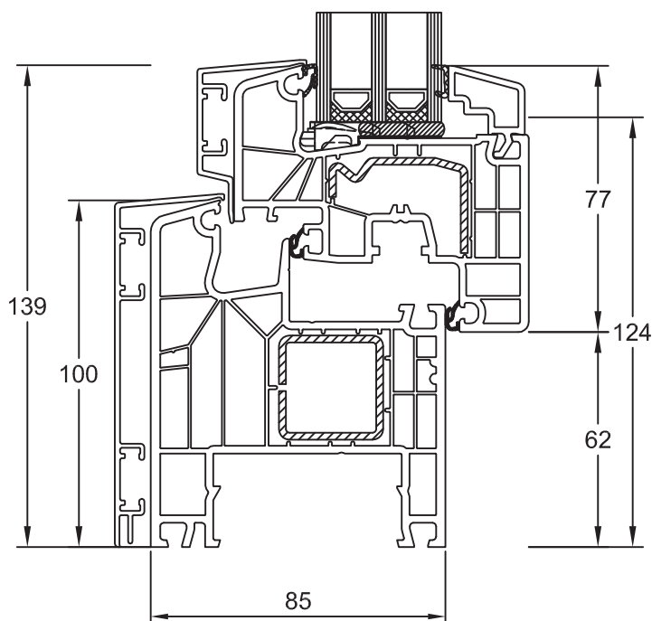
Blendrahmen 180x04/ S12630 Flügel Classic 180x20/ S12631
