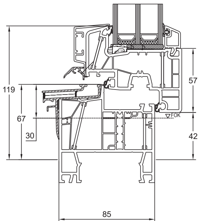
Blendrahmen 080x04 Flügel Classic 080x20 Einlegeschwelle
