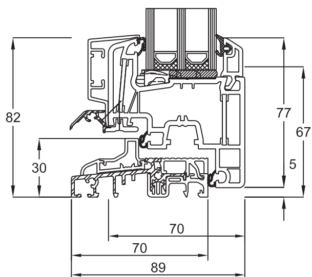
Bodenschwelle 249060 Adapter 287062 Flügel Classic 050x20
