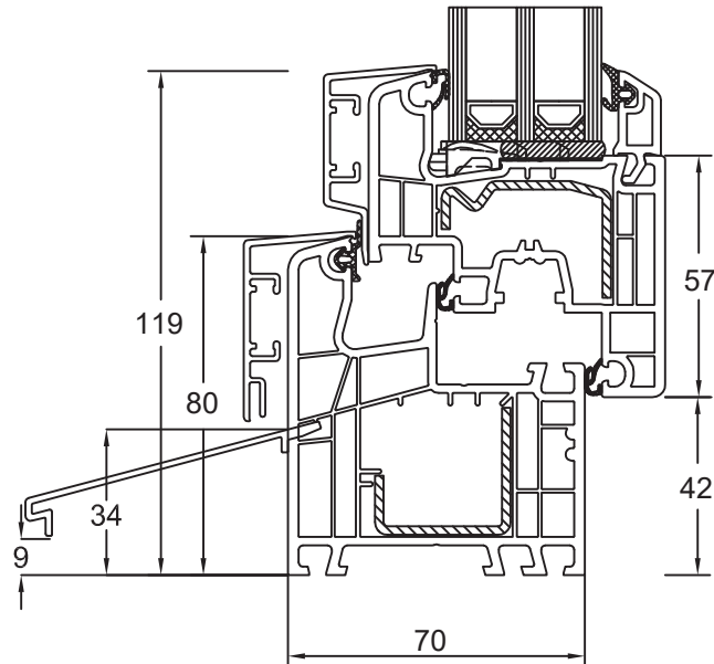
Blendrahmen 150x03 Flügel Classic 150x20 Wetterschenkel S12833
