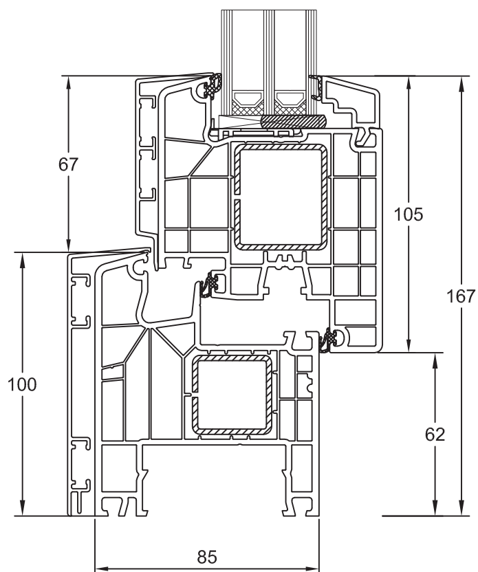
Blendrahmen 180x04/ S12630 Flügel Classic 180x20/ S12638
