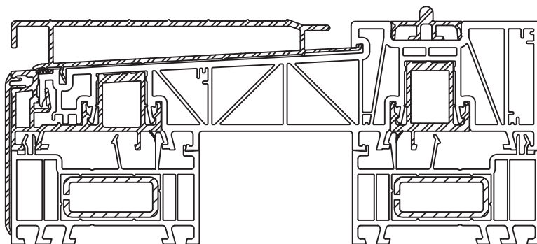
Schwelle STANDARD /PVC + ALU / barrierefrei + Trittschutz 277202 + Abschlussleiste 277206
