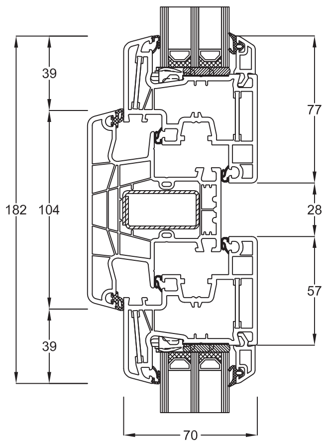
Pfosten 150x44 Flügel Classic 050x20
