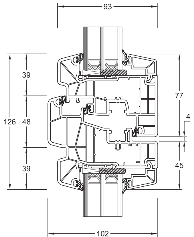
Stulpflügel 180x+69 Flügel hfv+ 8mm 180x26
