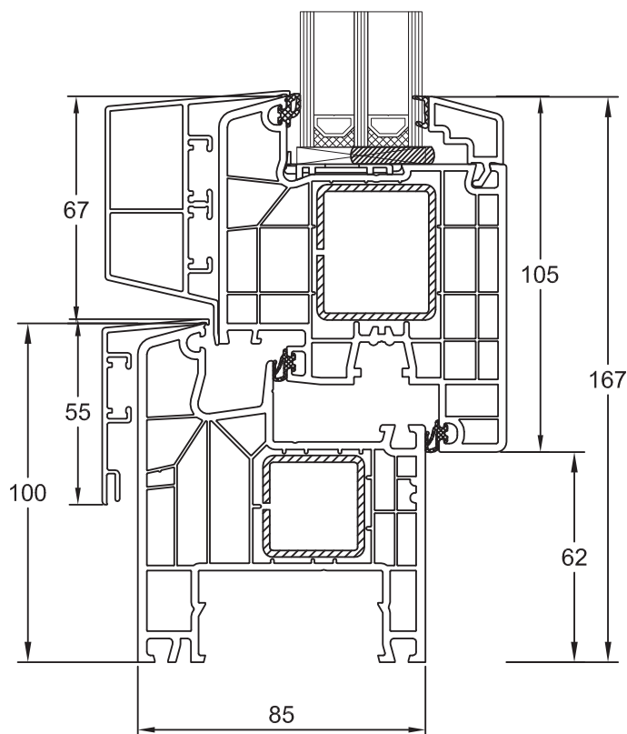
Blendrahmen 180x04/ S12630 Flügel Classic 180x30/ S12640
