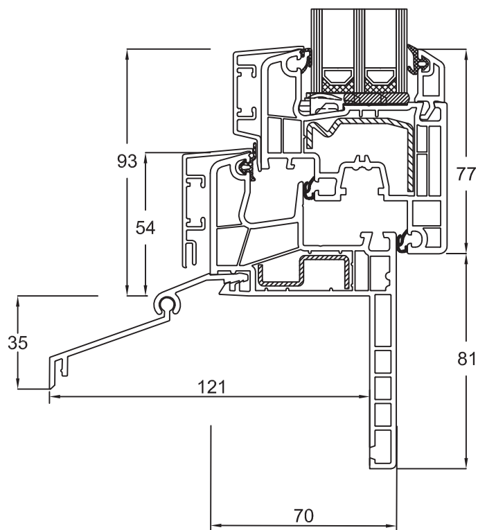
Blendrahmen 150x10 Flügel Classic 150x20 Kombiwetterschenkel VS4475+S13081
