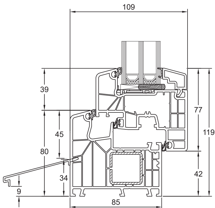
Blendrahmen 180x05 Flügel Classic 180x20 Wetterschenkel VS10995
