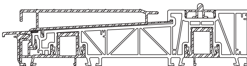
Schwelle STANDARD /PVC + ALU / barrierefrei + Trittschutz 277202 + Abschlussleiste 277205
