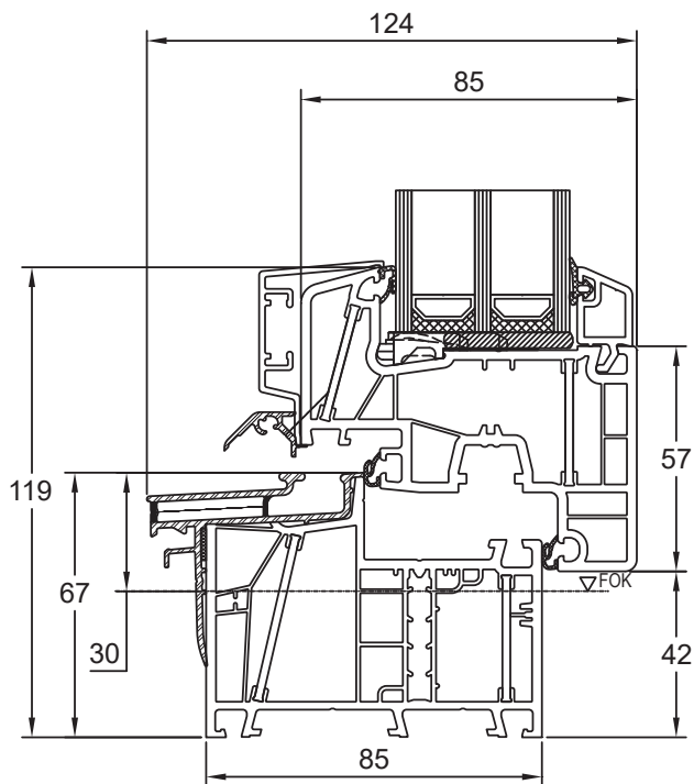
Blendrahmen 080x05 Flügel Classic 080x20 Einlegeschwelle
