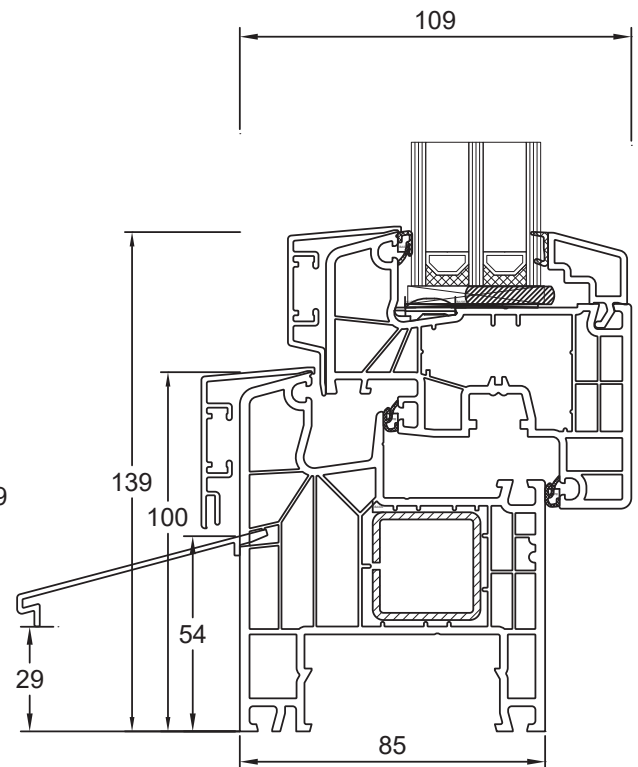
Blendrahmen 180x04/ S12628 Flügel Classic 180x20/ S12639 Wetterschenkel S12833
