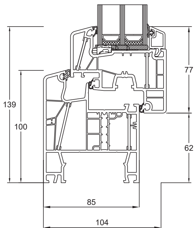
Blendrahmen 080x04 Flügel Classic 080x20
