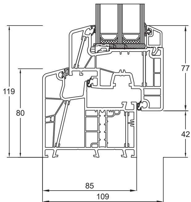
Blendrahmen 080x05 Flügel Classic 080x20
