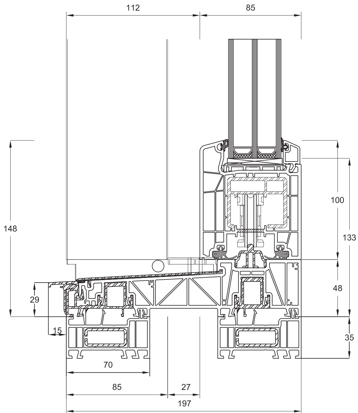
Schwelle Standard 277260 Flügel 170x81 STV 140205
