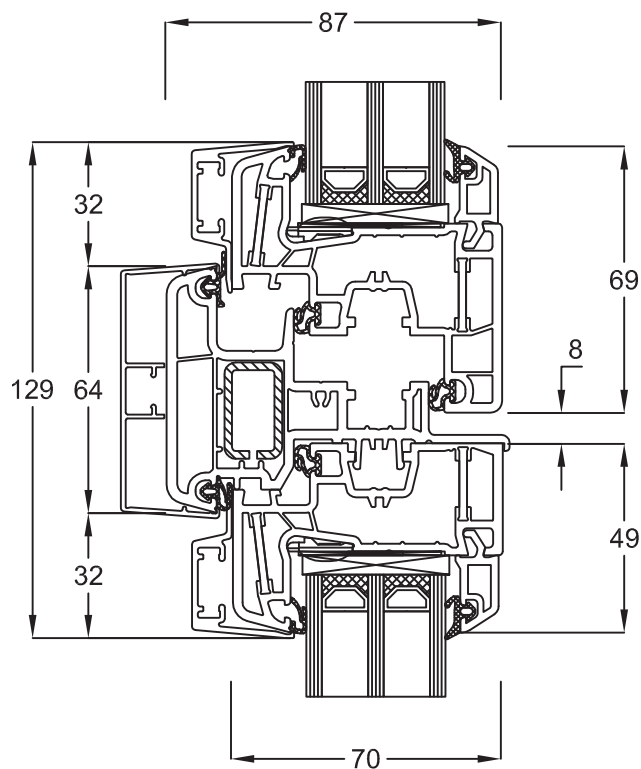
Stulp 150x65 Flügel Classic 050x24
