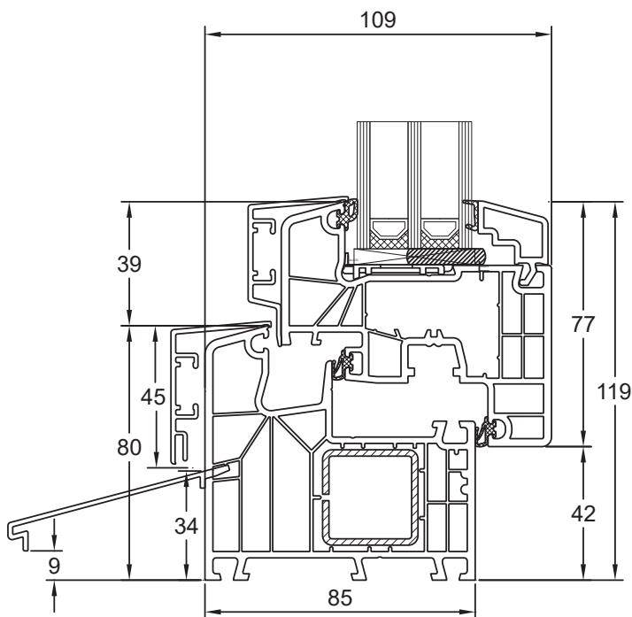
Blendrahmen 180x05/ S12628 Flügel Classic 180x20/ S12639 Wetterschenkel S12833
