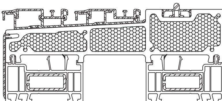
Schwelle PREMIUM / GFK / barrierefrei + Trittschutz 277107/277106 + Abschlussleiste 277206
