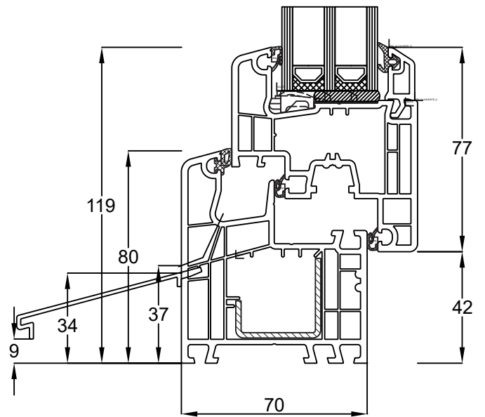
Blendrahmen 150x03 Flügel Classic 150x20 Wetterschenkel S12833
