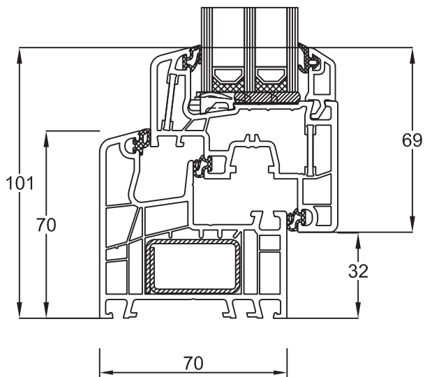
Blendrahmen 150x02 Flügel Classic 050x24
