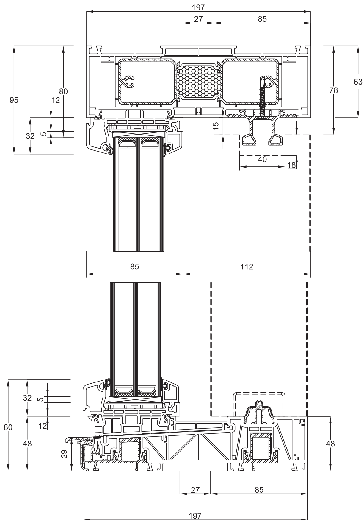
Schwelle STANDARD 277260 +Abschlussleiste277205 Flügel FIXFRAME 170082
