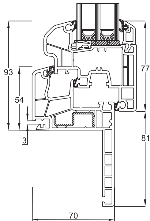
Blendrahmen 150x10 Flügel Classic 050x26
