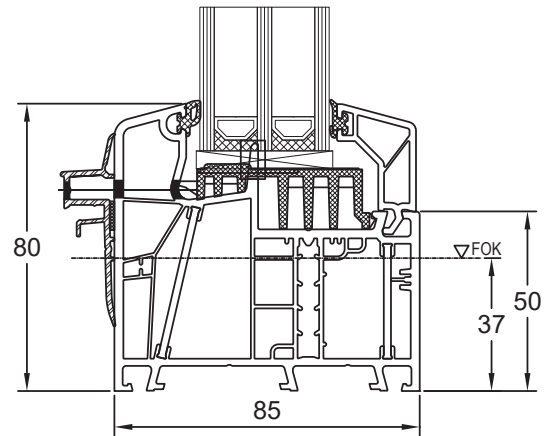
Blendrahmen 080x05 Einlegeschwelle FIX
