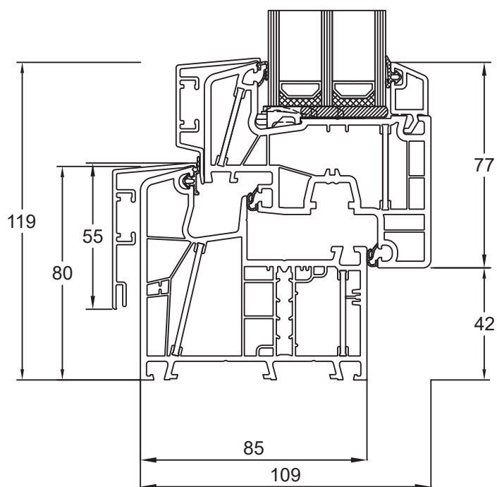
Blendrahmen 080x05 Flügel Classic 080x20
