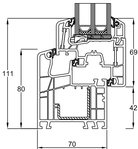
Blendrahmen 150x03 Flügel 050x24
