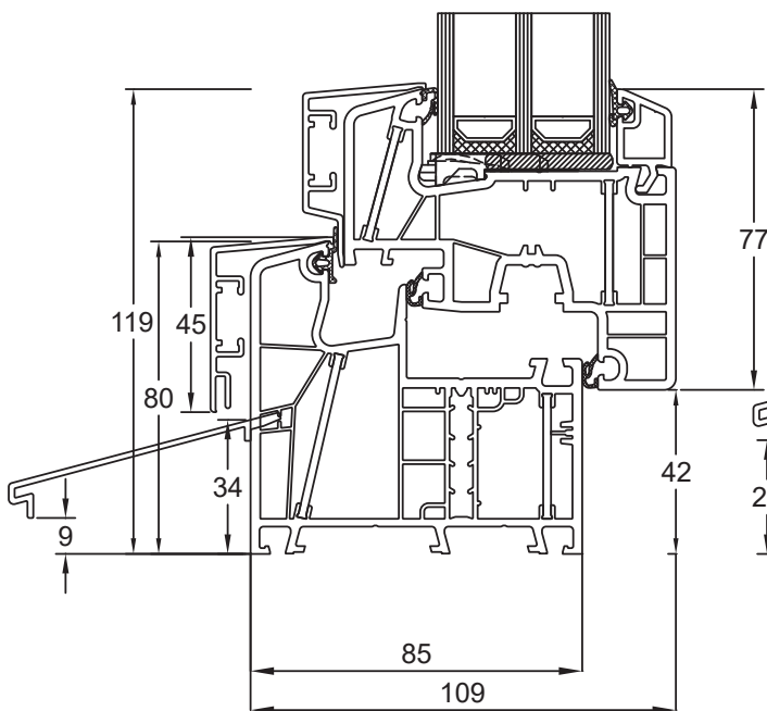
Blendrahmen 080x05 Flügel Classic 080x20 Wetterschenkel S12833
