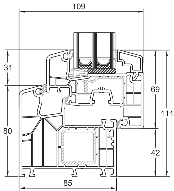
Blendrahmen 180x05 Flügel Classic 180x24
