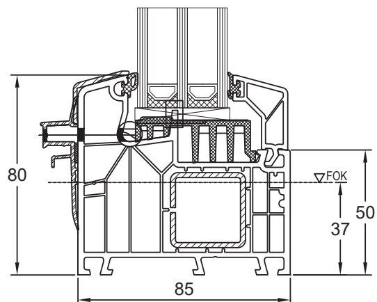
Blendrahmen 180x05 Einlegeschwelle FIX
