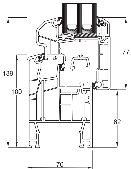
Blendrahmen 050x04 Flügel hfv 150x26
