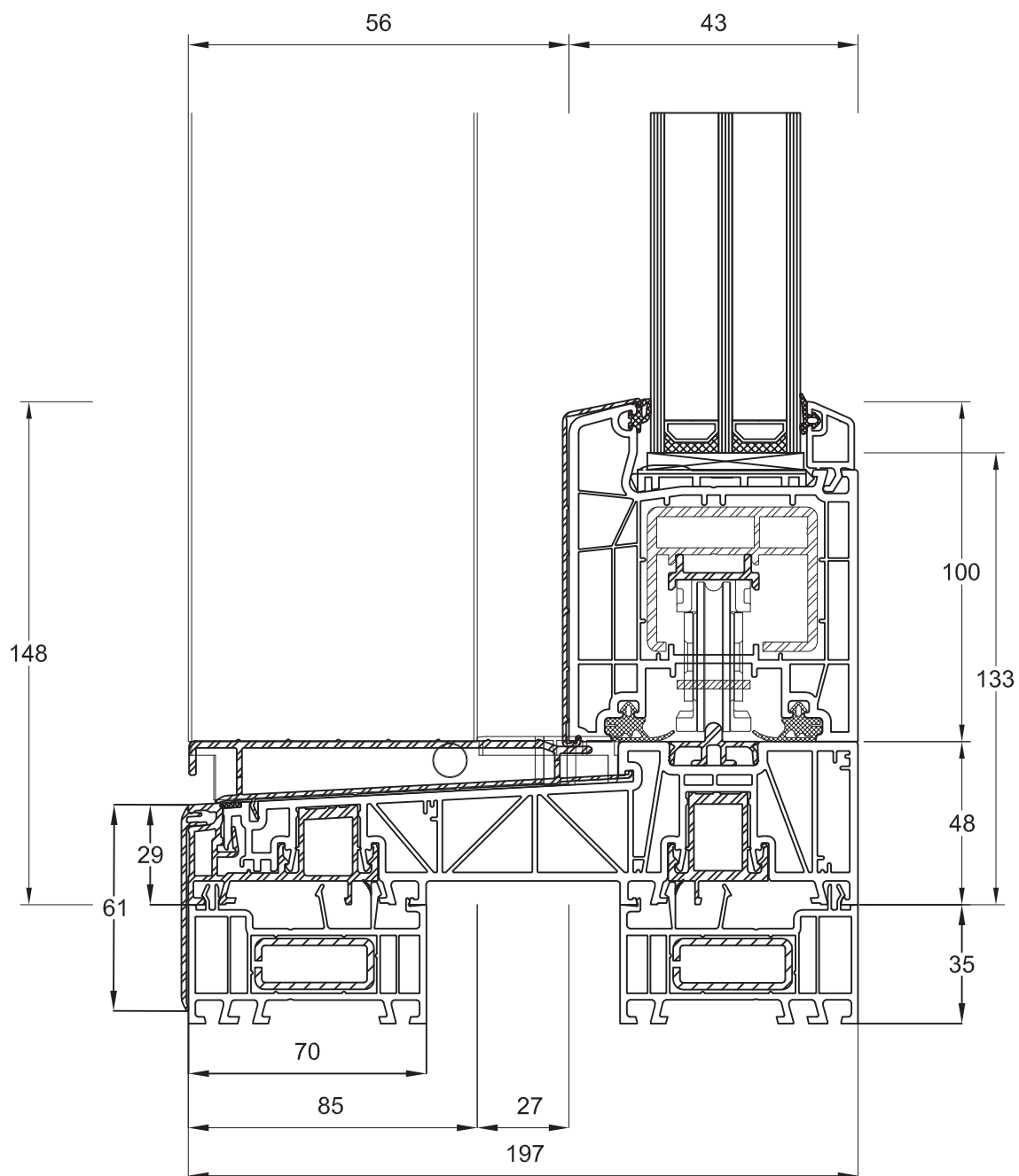
Schwelle Standard 277260 Flügel 170x81 STV 140205 ALU Abschlussleiste 277210 Trittschutz berrierefrei 277202
