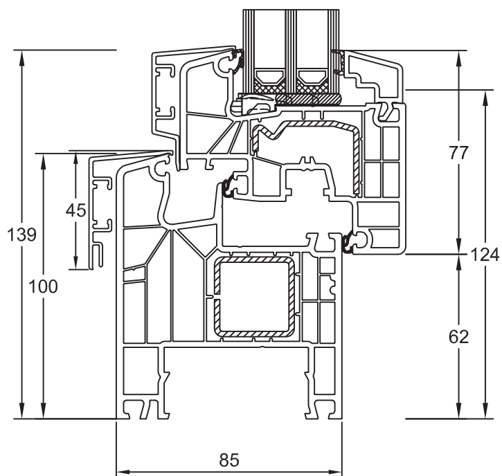
Blendrahmen 180x04/ S12628 Flügel Classic 180x20/ S12631
