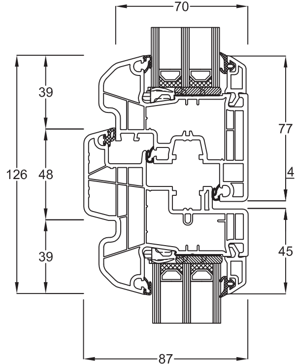
Stulpflügel 150x69 Flügel hfv 150x26
