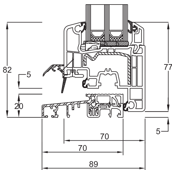
Bodenschwelle 249060 Flügel Classic 150x20
