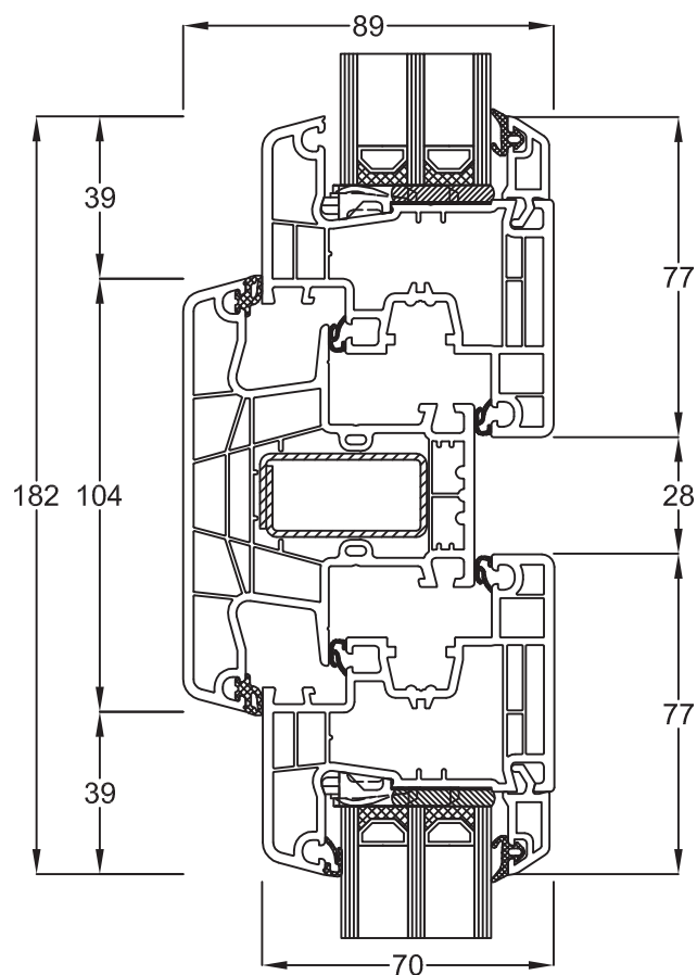
Pfosten 150x44 Flügel Classic 150x20
