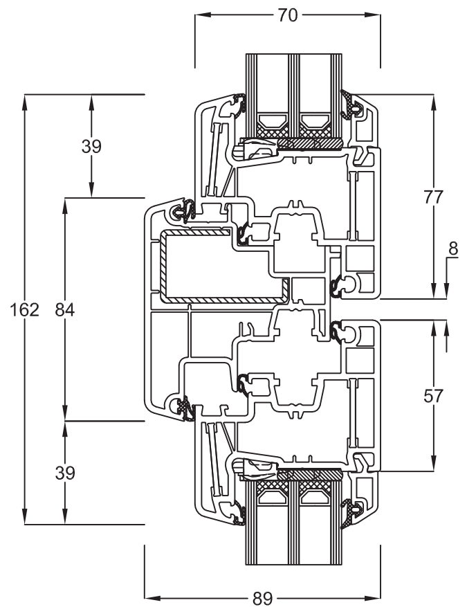
Stulp 150x67 Flügel Classic 050x24
