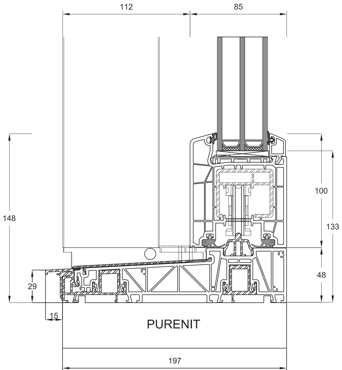
Schwelle Standard 277260 Flügel 170x81
