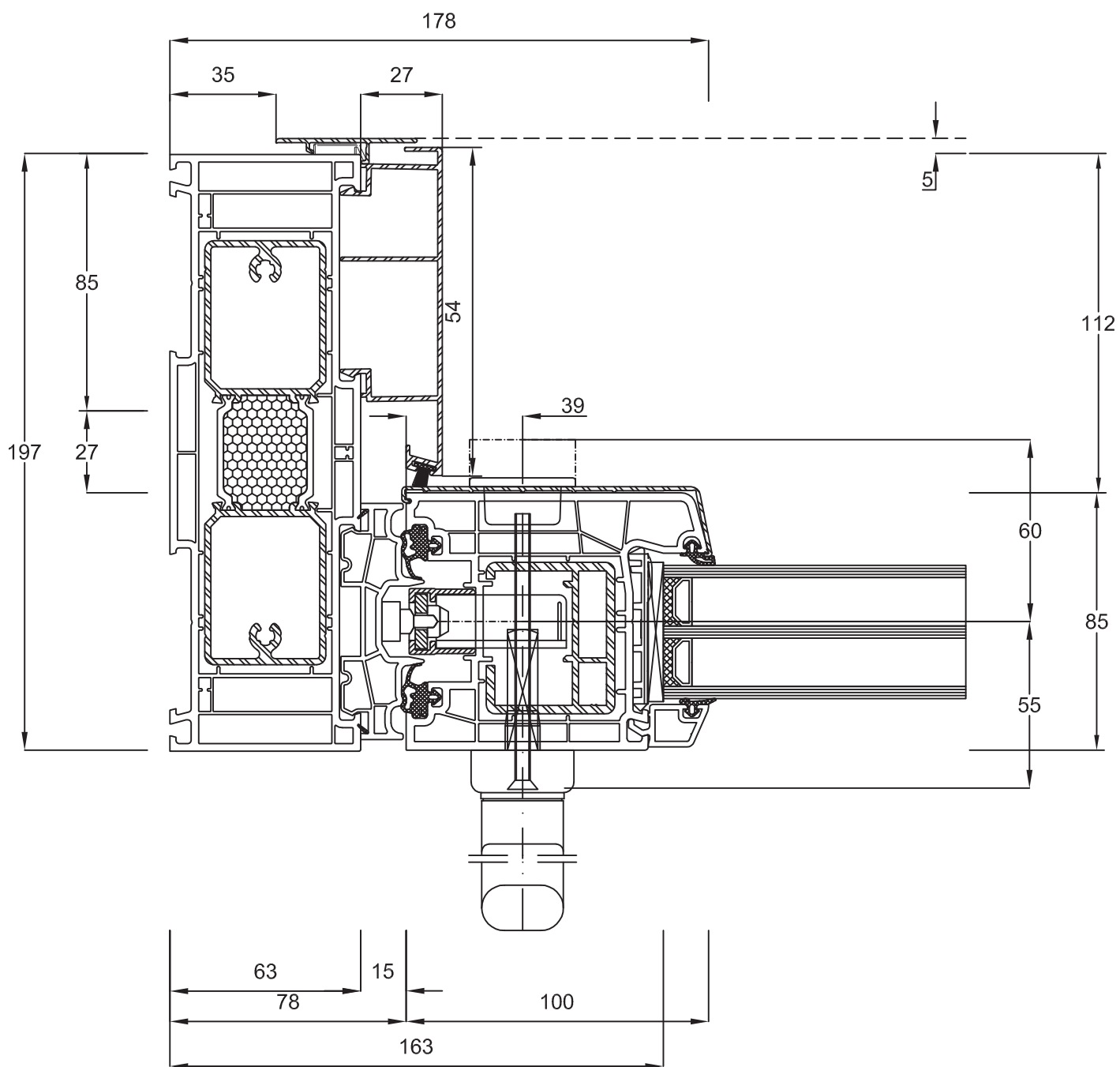
Zarge 170080 Flügel 170x81 Aluprotect Zarge kurz
