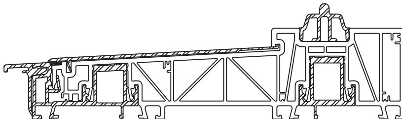
Schwelle STANDARD / PVC+ALU / mit Trittschutz 277201 + Abschlussleiste 277205
