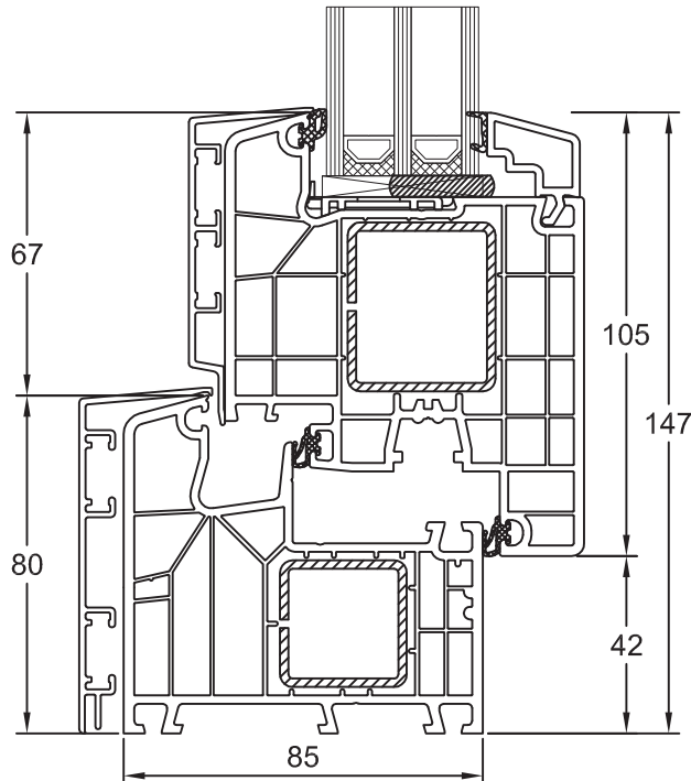
Blendrahmen 180x05/ S12929 Flügel Classic 180x20/ S12631
