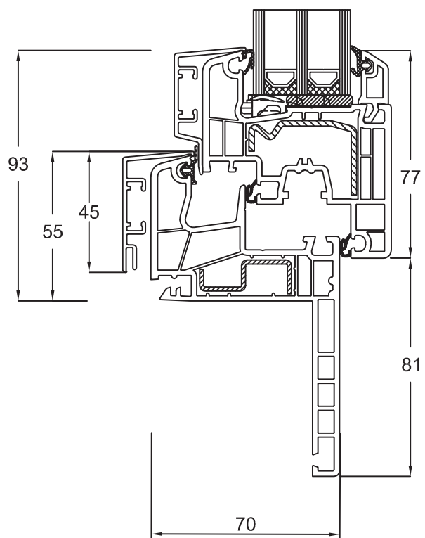
Blendrahmen 150x10 Flügel Classic 150x20
