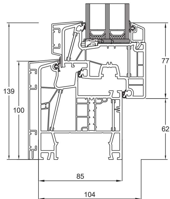
Blendrahmen 080x04 Flügel Classic 080x20
