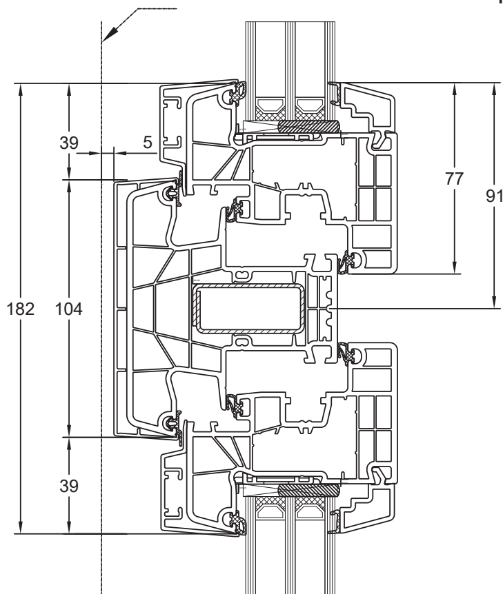
Pfosten 180x44 Flügel Classic 180x20
