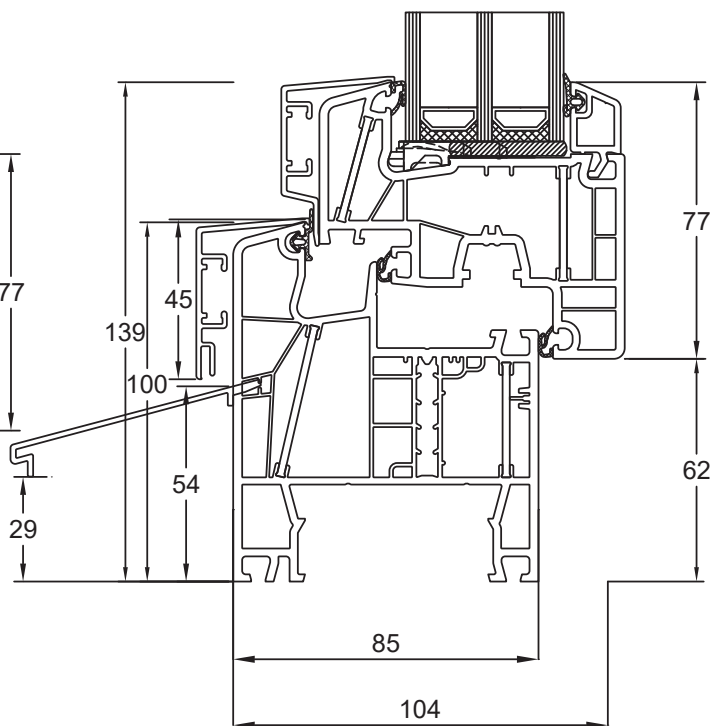
Blendrahmen 080x04 Flügel Classic 080x20 Wetterschenkel S102833
