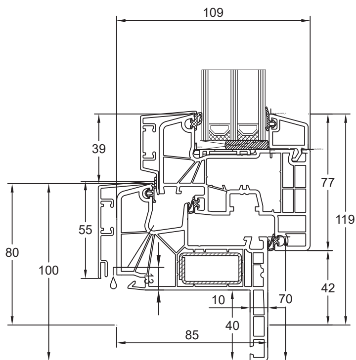
Blendrahmen 180x15 Flügel Classic 180x20
