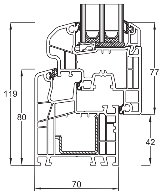
Blendrahmen 150x03 Flügel hfv 150x26
