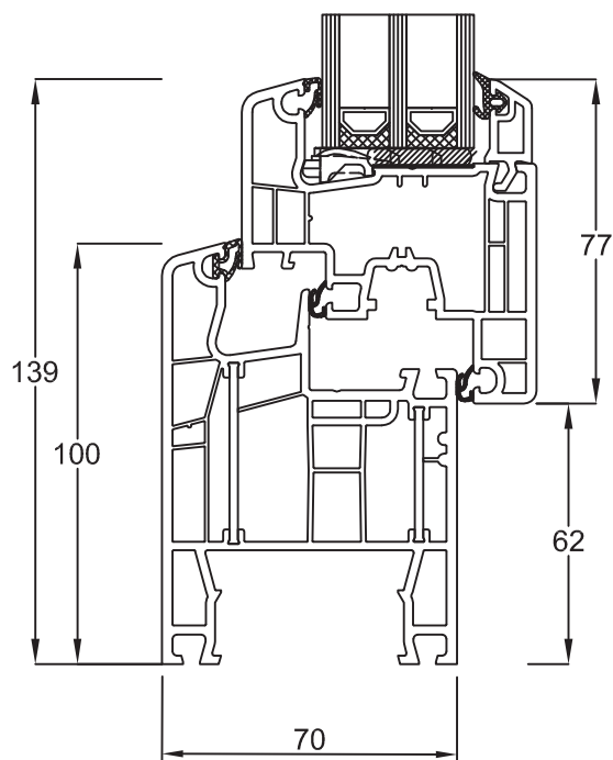
Blendrahmen 050x04 Flügel Classic 150x20
