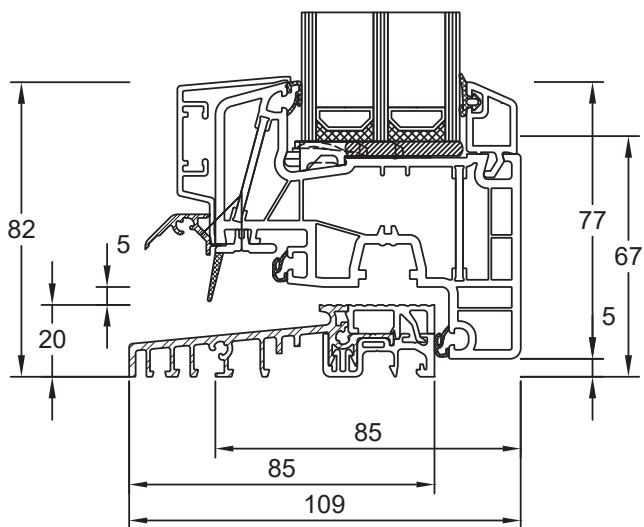
Flügel Classic 080x20 Bodenschwelle 269060
