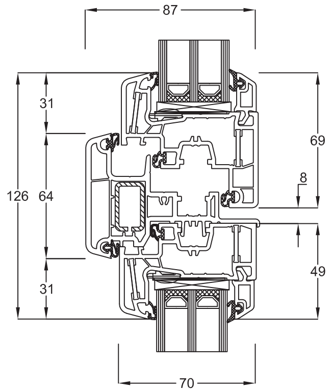
Stulp 150x65 Flügel Classic 050x24
