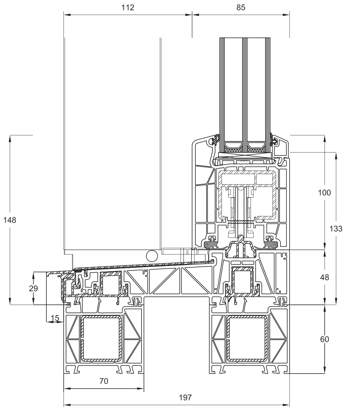
Schwelle Standard 277260 Flügel 170x81 STV 140207
