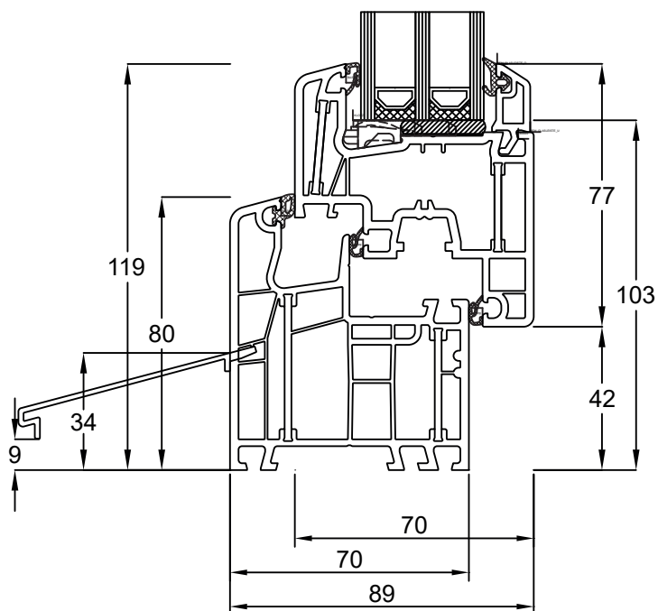
Blendrahmen 050x03 Flügel Classic 050x20 Wetterschenkel S12833
