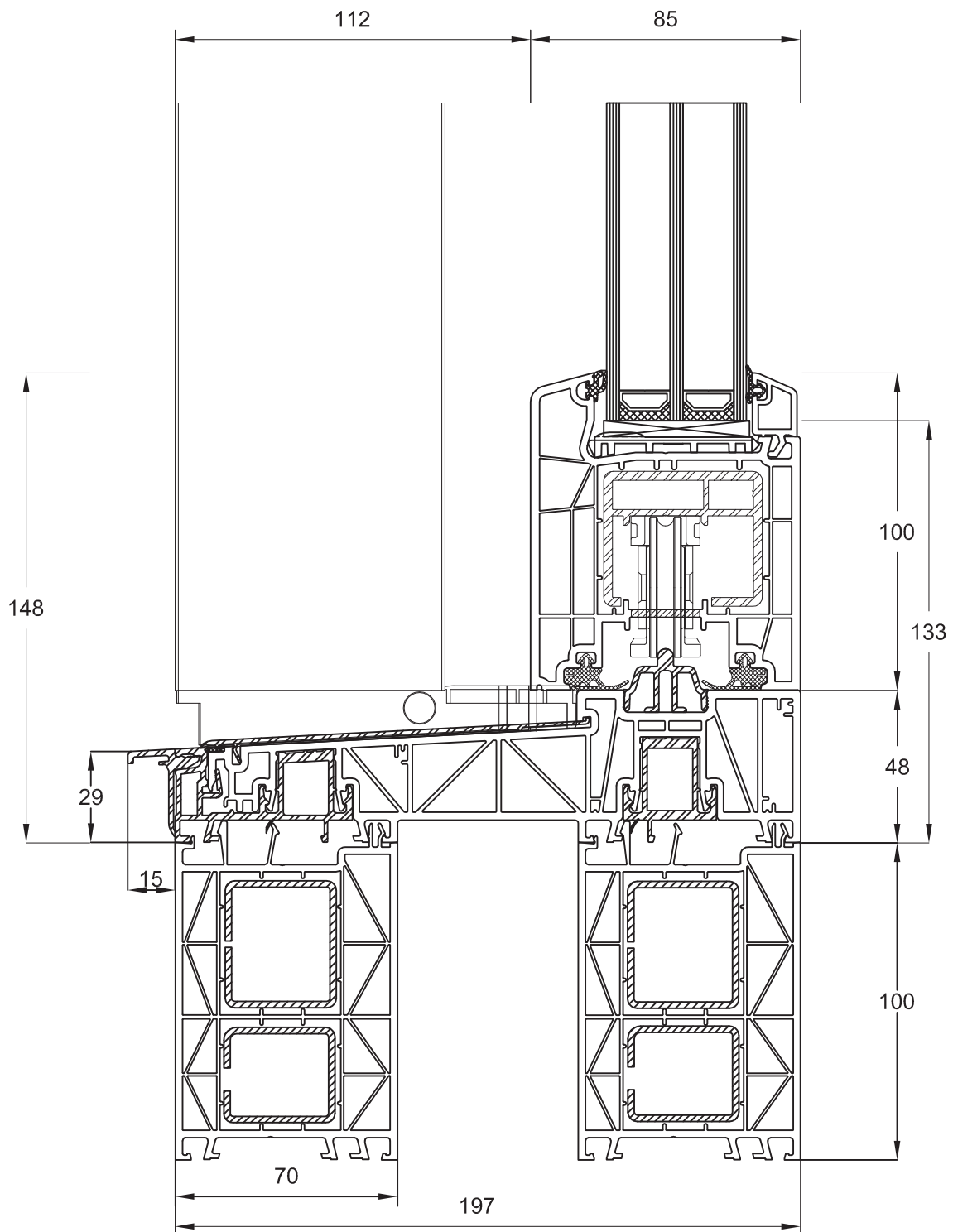
Schwelle Standard 277260 Flügel 170x81 STV 140208
