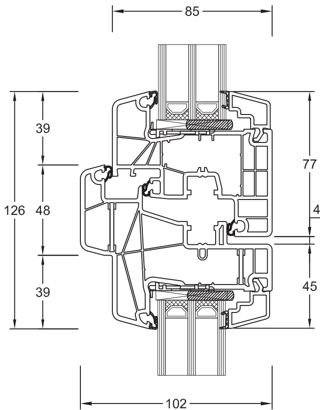
Stulpflügel 080x89 Flügel Classic 180x20
