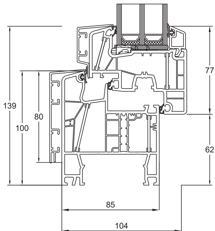
Blendrahmen 080x04 Flügel Classic 080x20
