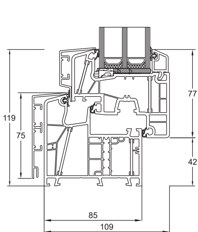
Blendrahmen 080x05 Flügel Classic 080x20
