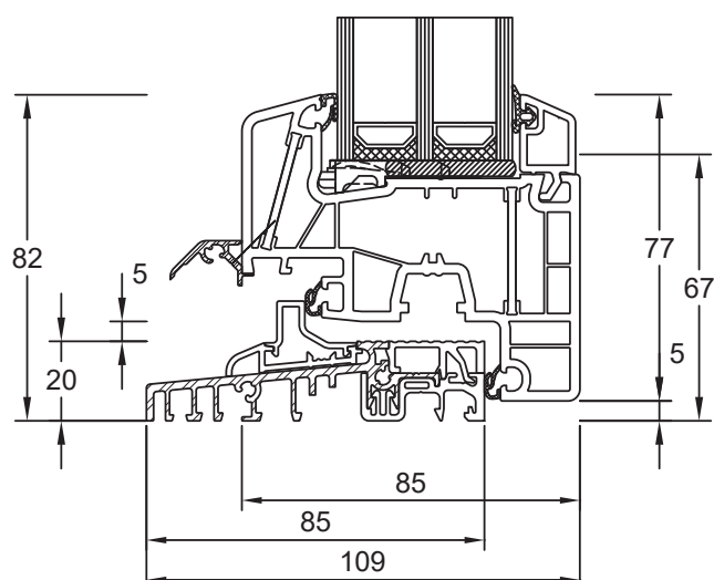
Flügel Classic 080x20 Bodenschwelle 269060 Schwellenadapter 287062
