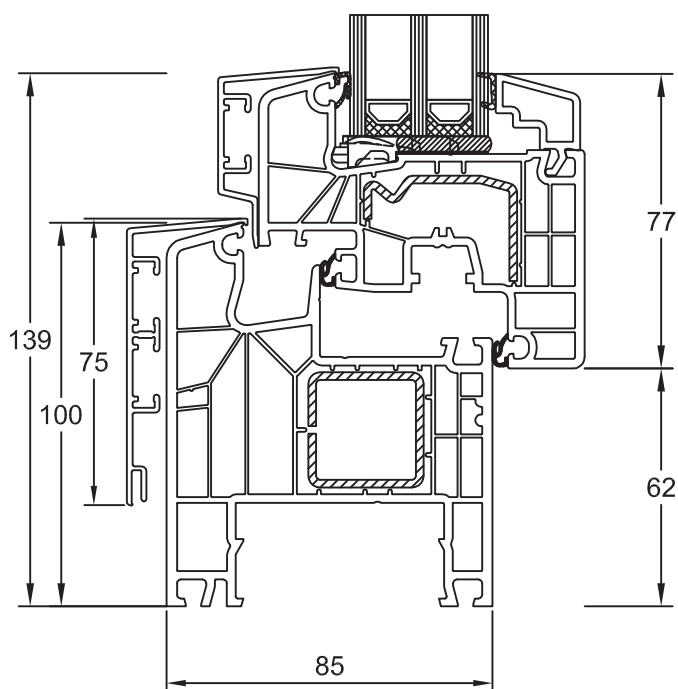
Blendrahmen 180x04/ S12694 Flügel Classic 180x20/ S12631
