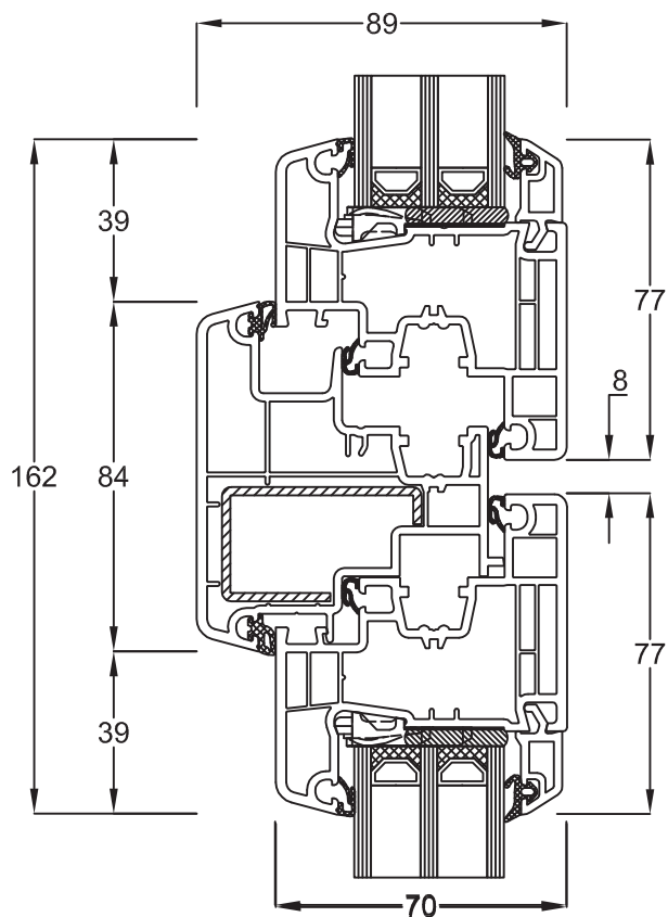
Stulp 150x67 Flügel Classic 150x20
