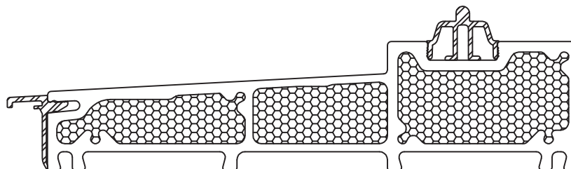
Schwelle PREMIUM / GFK /+ Abschlussleiste 277205
