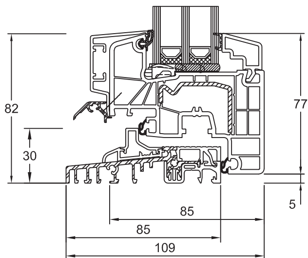
Flügel Classic 180x20/ S12631 Bodenschwelle 269060 Schwellenadapter 287062
