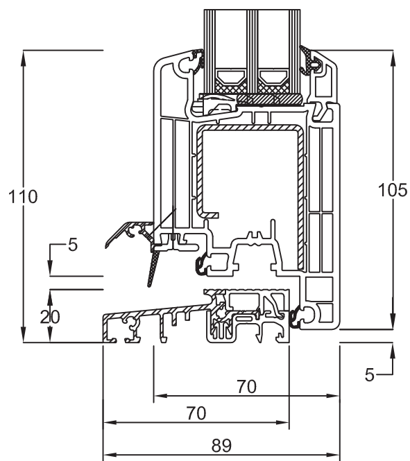
Bodenschwelle 249060 Flügel Classic 150x30
