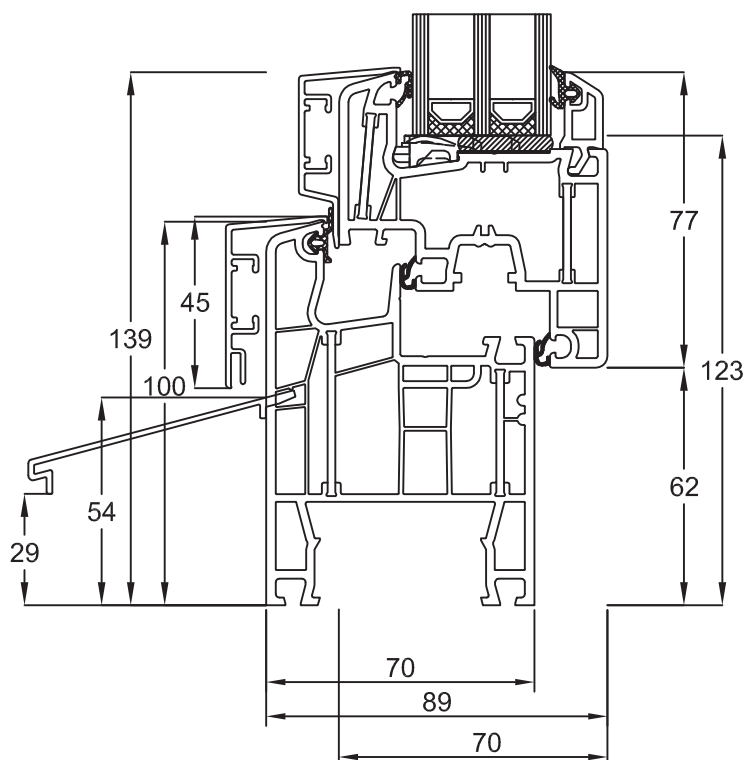
Blendrahmen 050x04 Flügel Classic 050x20 Wetterschenkel S12833
