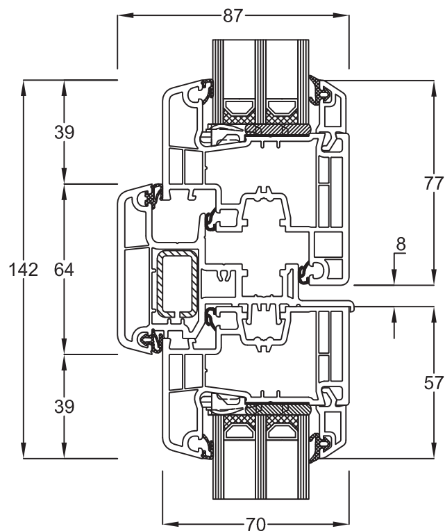
Stulp 150x65 Flügel 150x20
