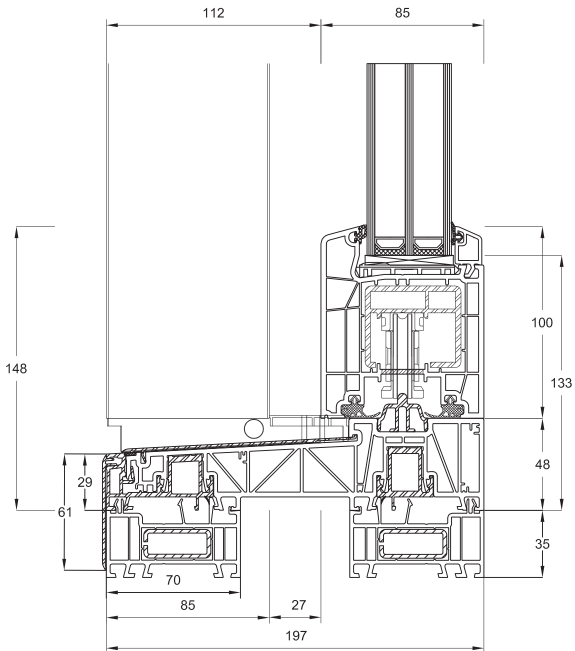
Schwelle Standard 277260 Flügel 170x81 STV 140205 ALU Abschlussleiste 277210
