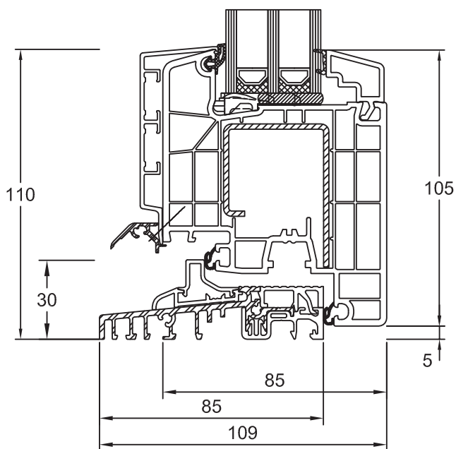
Flügel Classic 180x30/ S12638 Bodenschwelle 269060 Schwellenadapter 287062
