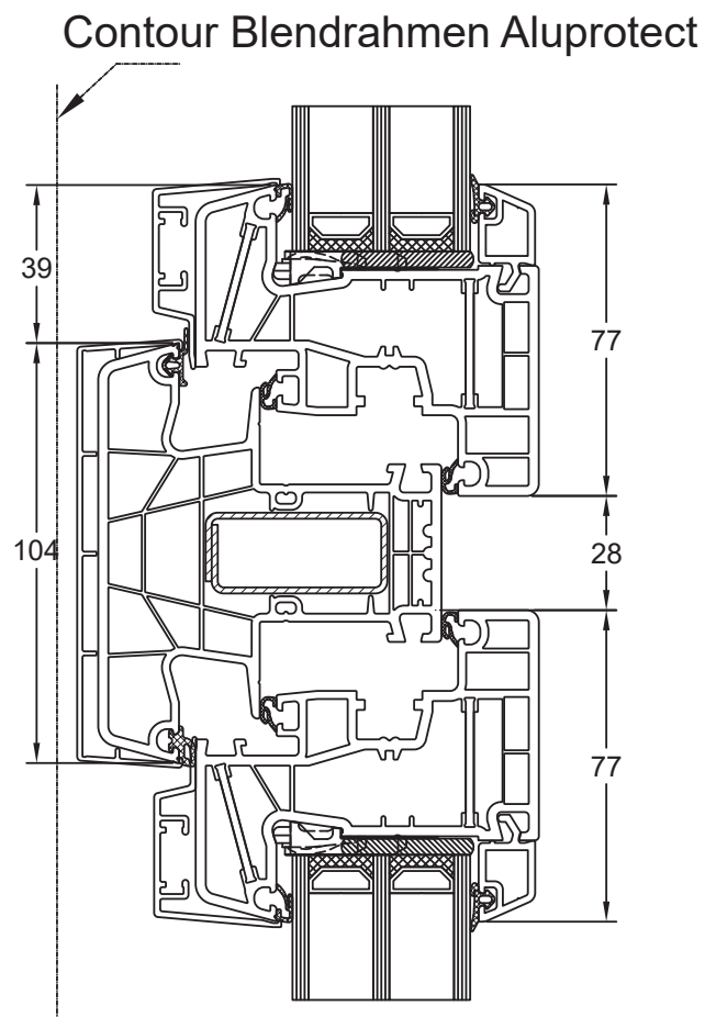
Pfofen 180x44 Flügel Classic 080x20
