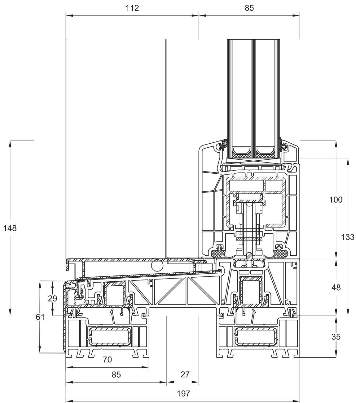
Schwelle Standard 277260 Flügel 170x81 STV 140205 ALU Abschlussleiste 277210 Trittschutz barrierefrei 277202
