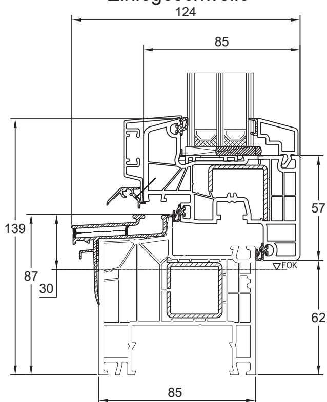
Blendrahmen 180x05 Flügel Classic 180x20 Einlegeschwelle
