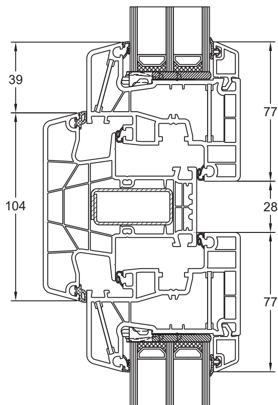
Pfosten 180x44 Flügel Classic 080x20
