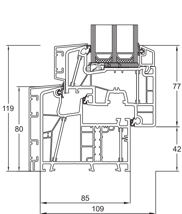
Blendrahmen 080x05 Flügel Classic 080x20
