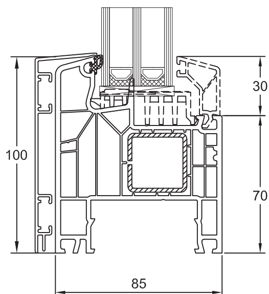
Blendrahmen 180x04/ S12630
