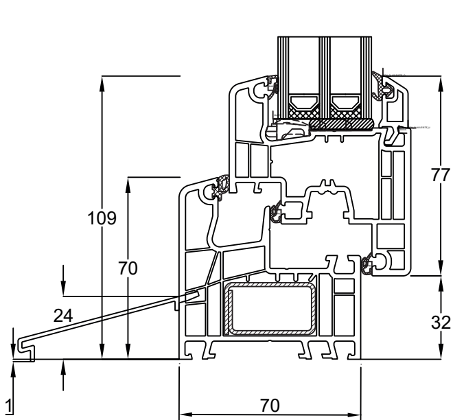
Blendrahmen 150x02 Flügel Classic 150x20 Wetterschenkel S12833
